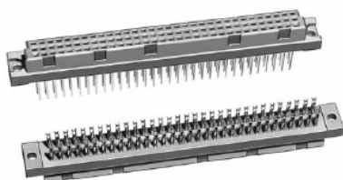
DIN 41612 TIPO C
